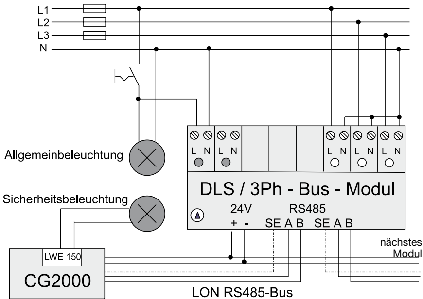
Bild 3: Schaltung eines DLS/3PH BUS-Moduls
