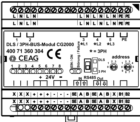
Bild 1 Anschlussbild DLS/3PH Modul
