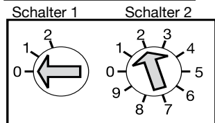
Bild 7 Adressschalter (nur STYLE 22011 CG)
